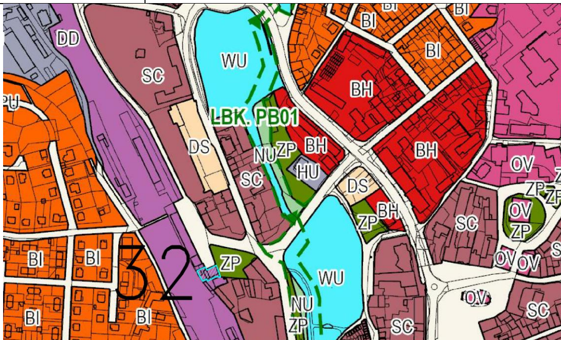
Hlavní výkres
